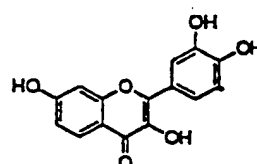
FISETIN
